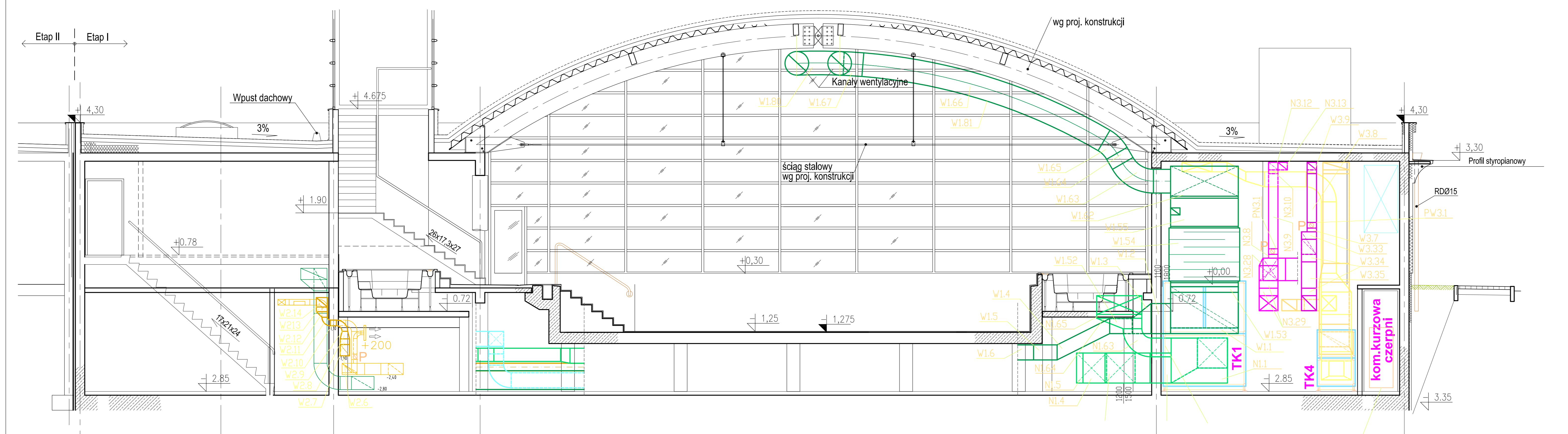
PRZEKRÓJ 3'-3'
